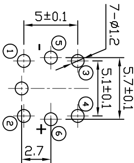
P.C.B LAYOUT
